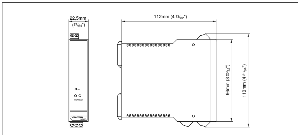
Рис. 7: Размеры VEGATRENN 149A Ex
