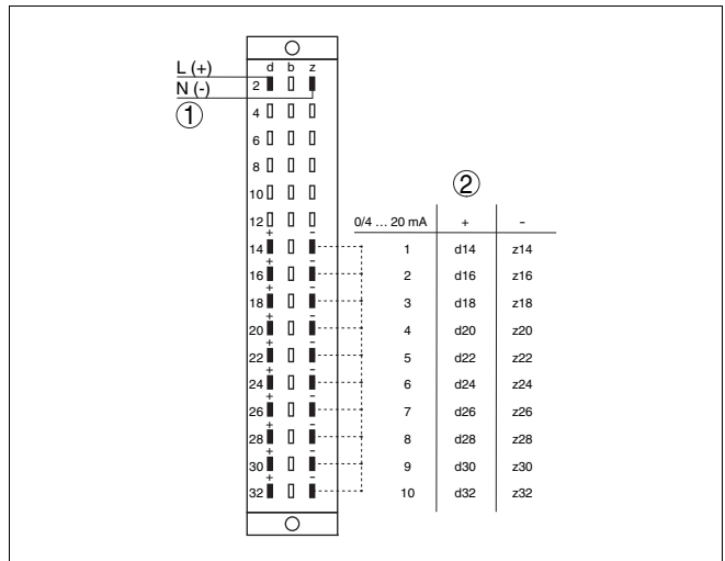
Fig. 3: VEGALOG 571 AA 1)
