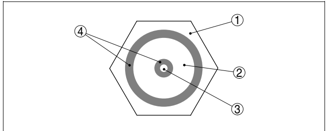
Fig. 2: Electrodo anular
