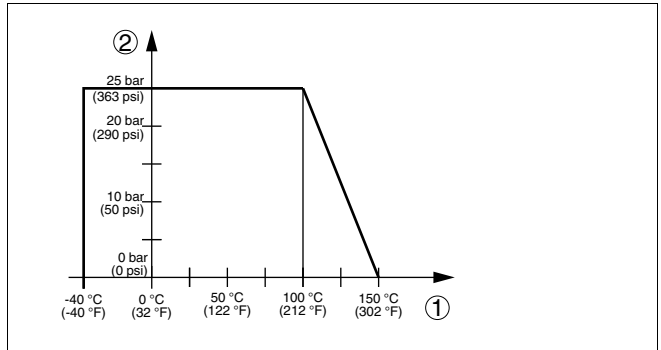
Fig. 22: Presión proceso - Temperatura de proceso
