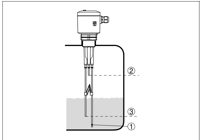
Abb. 2: Funktionsprinzip
