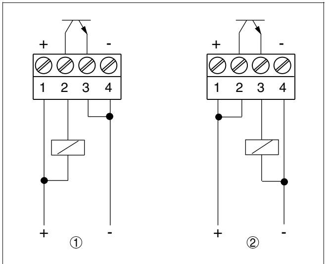
Abb. 6: Elektronik mit Transistorausgang
