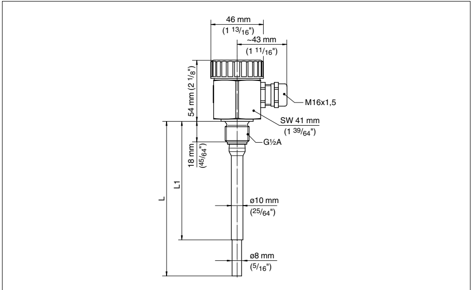
Fig. 8: Sonde de mesure résistive à tige EL 1
