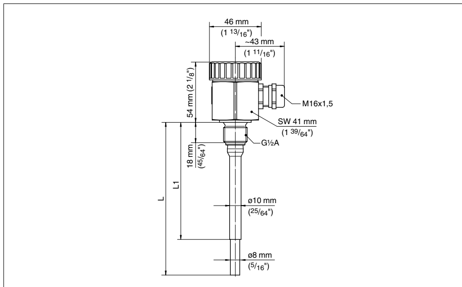
Fig. 8: Sonda condutiva de medição com haste EL 1
