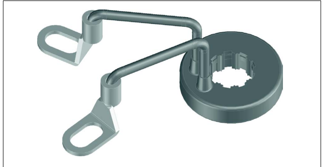
Fig. 6: Componente para a monitoração da fiação em combinação com o VEGATOR 632
