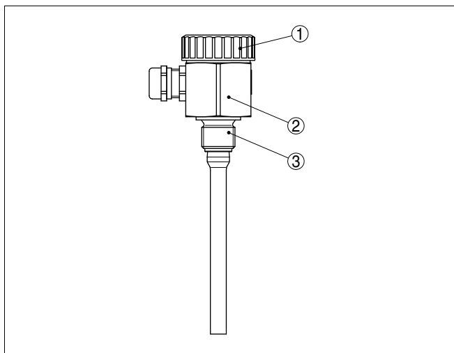
Fig. 1: Sonda condutiva de medição com haste EL 1
