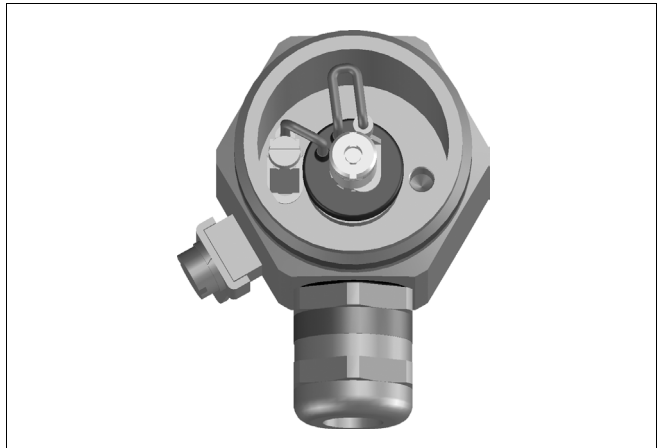
Fig. 7: Montagem do componente para a monitoração da fiação
