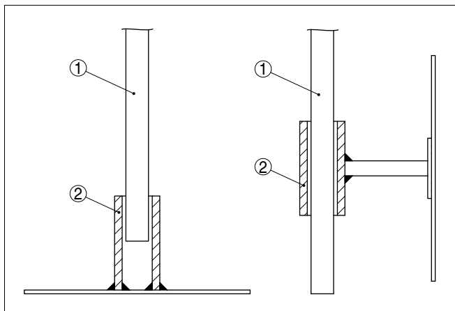
Fig. 3: Fixer la sonde de mesure
