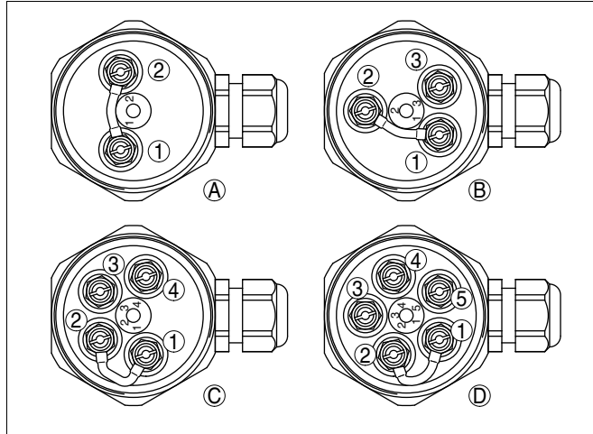
Fig. 5: Compartiment de raccordement de la sonde - résistance 220 k \Omega entre les bornes 1 et 2
