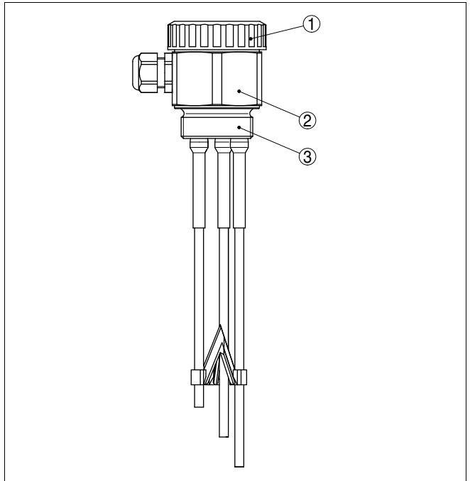
Fig. 1: Sonde de mesure résistive à plusieurs tiges EL 3
