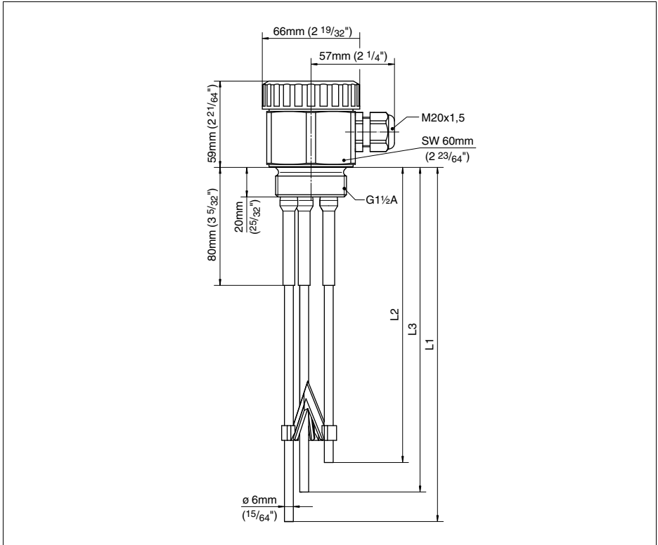
Fig. 8: Sonde de mesure résistive à plusieurs tiges EL 3
