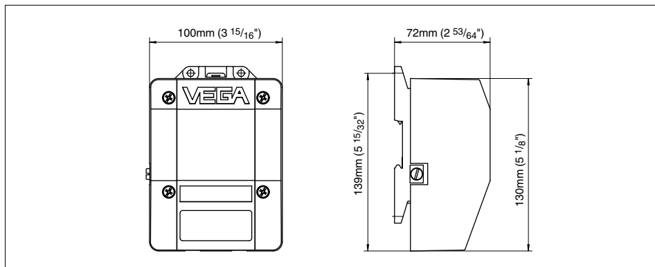
Рис. 8: VEGABOX 02 с защитным колпаком
