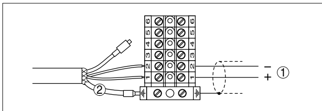
Рис. 3: Схема расположения контактов VEGABOX 02
