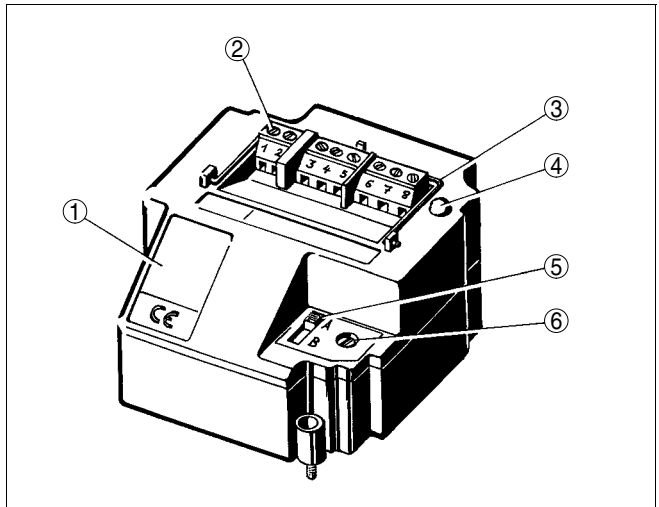
Fig. 6: Sistema eletrônico com saída de relê
