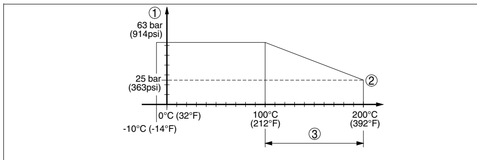
Fig. 21: Pressão do processo - temperatura do processp - VEGACAP 27 com conexão do processo de 316L
