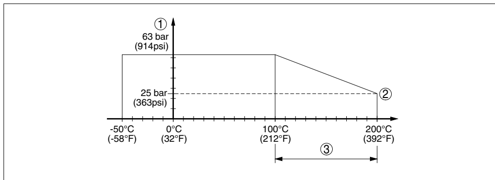
Fig. 22: Pressão do processo - temperatura do processp - VEGACAP 27 com conexão do processo de 316Ti
