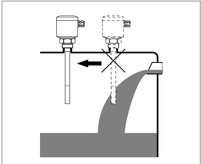
Abb. 4: Einströmendes Füllgut
