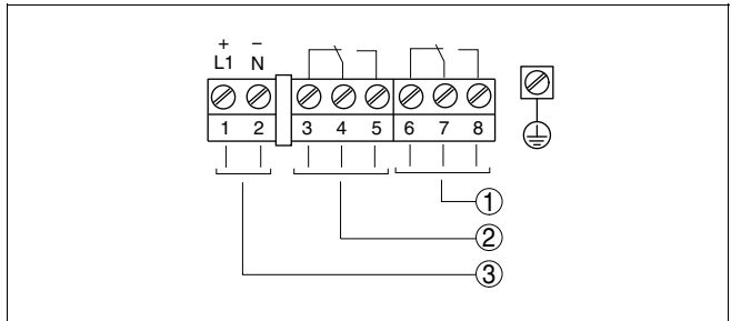
Abb. 5: Anschlussplan
