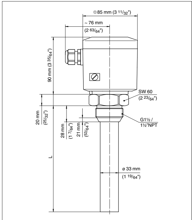
Abb. 24: VEGACAP 98, Gewindeausführung G1 1/2 A L = Sensorlänge, siehe Kapitel "Technische Daten"
