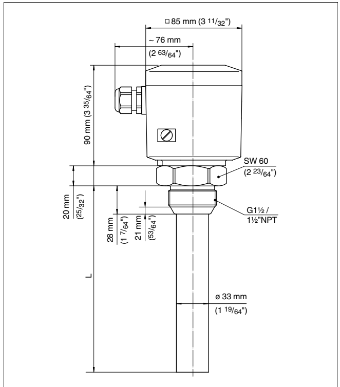
Fig. 24: VEGACAP 98, Versión roscada G1\frac{1}{2} A
