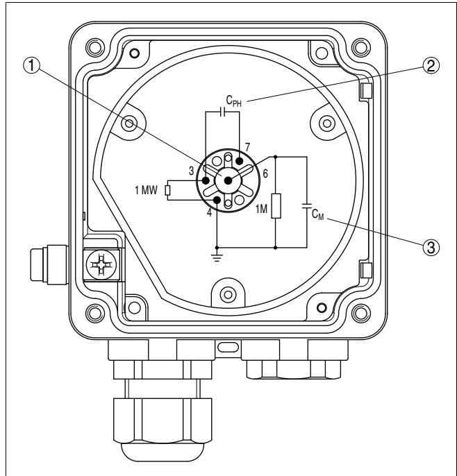
Fig. 21: Verificar a resistência dentro da sonda de medição
