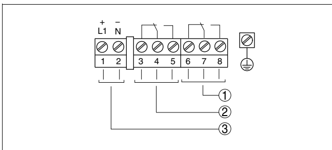
Fig. 5: Esquema de ligações
