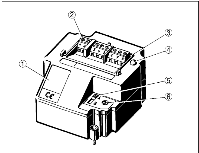
Fig. 6: Sistema eletrônico com saída de relê
