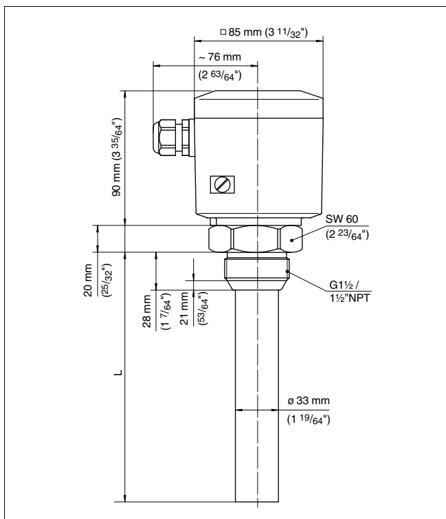
Fig. 22: VEGACAP 98, Modelo com rosca G1 1/2 A L = comprimento do sensor, vide "Dados técnicos"
