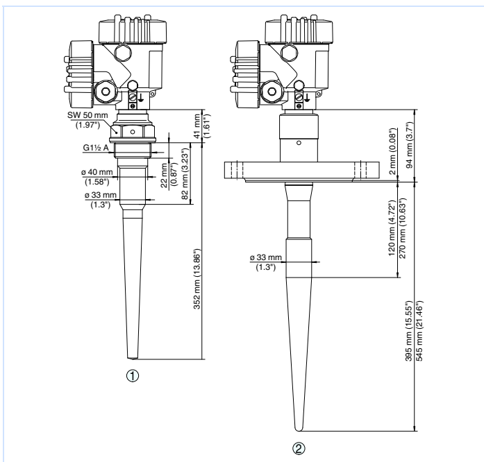
Dimensões do VEGAPULS 65
