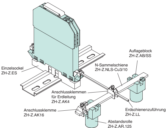
Abbildung 1.10 Isolierte Montage (Einzelerdung)
