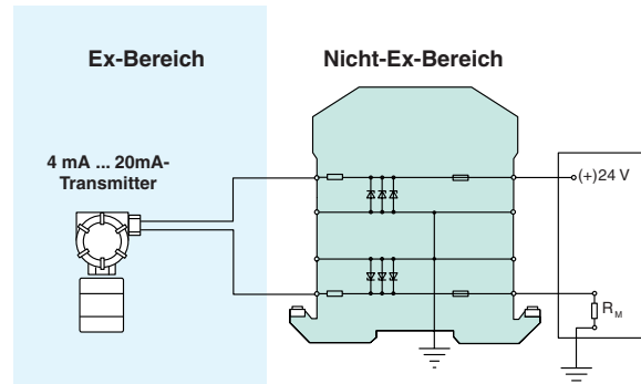
Abbildung 1.5 Zweikanalige Zenerbarriere
