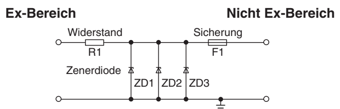
Abbildung 1.1 Prinzipschaltbild
