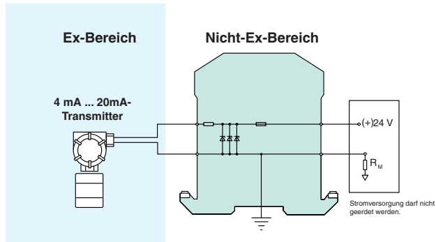
Abbildung 1.4 Einkanalige Zenerbarriere
