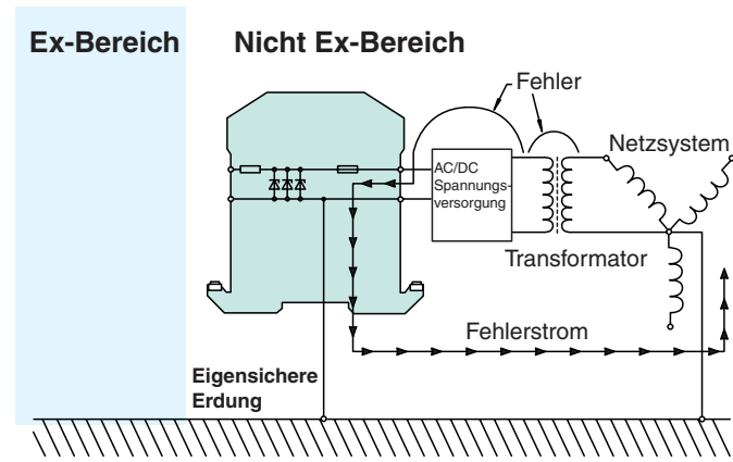
Abbildung 1.7 Geerdete Zenerbarriere
