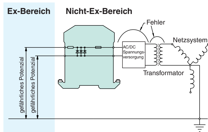
Abbildung 1.6 Nicht geerdete Zenerbarriere
