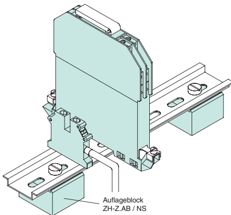
Abbildung 1.9 Isolierte Montage (Gruppenerdung)
