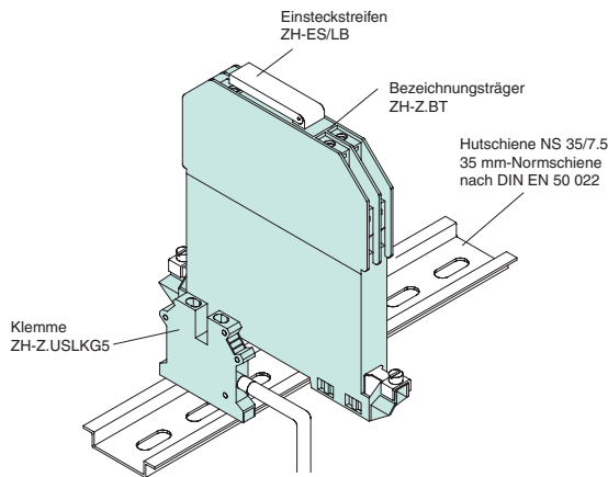
Abbildung 1.8 Potenzialausgleich über die Normschiene
