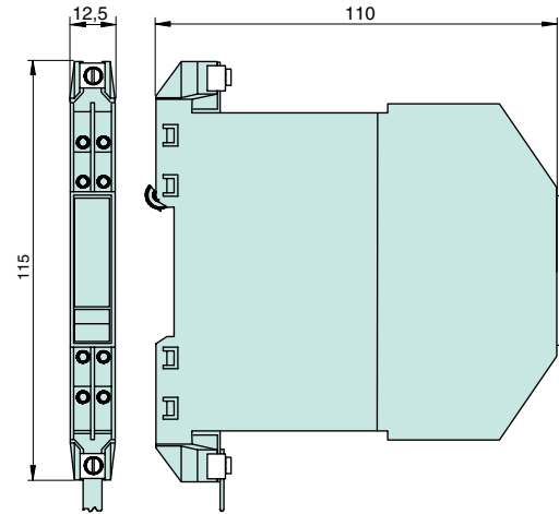
Abbildung 1.11 Mechanik
