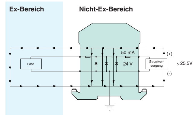
Abbildung 1.3 Diese Abbildung zeigt, dass beim Überschreiten der maximal zulässigen Eingangs-(Versorgungs-)Spannung der gesamte Strom durch die Zenerdioden abfließt, ohne die explosive Umgebung zu erreichen.
