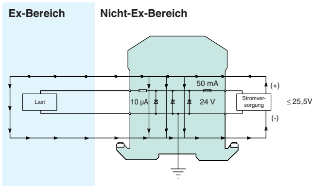
Abbildung 1.2 Diese Abbildung zeigt eine Auswahl an Leckströmen durch die Zenerbarrieren unter normalen Umständen. Die Zenerbarrieren leiten höchstens 10 (1) \mu\text{A} -Leckströme, solange die Versorgungsspannung unter 25,5 \text{ V} liegt. Das ist normal und hat wenig Einfluss auf die Last. Wenn die Spannung 25,5 \text{ V} überschreitet, beginnen die Zenerdioden mehr Strom zu leiten. Das kann den Laststrom und die Genauigkeit beeinflussen. Daher wird empfohlen, eine geregelte Spannungsquelle einzusetzen, welche die Spannung unter dem Wert hält, bei dem die Dioden zu leiten anfangen. (Zu Beispielszwecken wird eine 24 \text{ V} , 300 \text{ Ohm} -Barriere dargestellt.)
