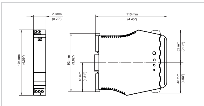
Medidas VEGATRENN 151
