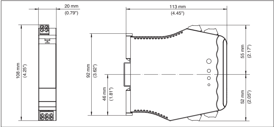
Fig. 3: Medidas VEGATRENN 152
