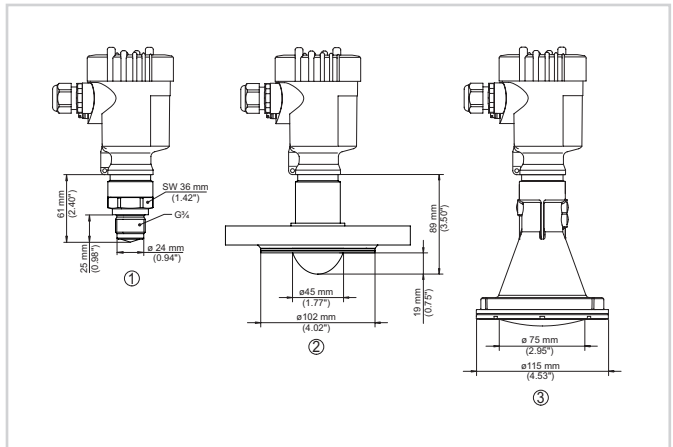
Dimensioni VEGAPULS 64
