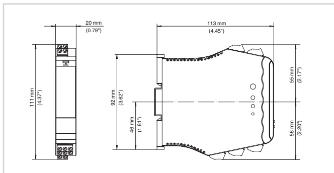
Medidas VEGATRENN 142
