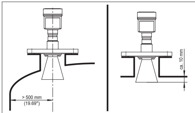
Fig. 1: Écarts de l'antenne à la paroi de la cuve/au couvercle de la cuve
