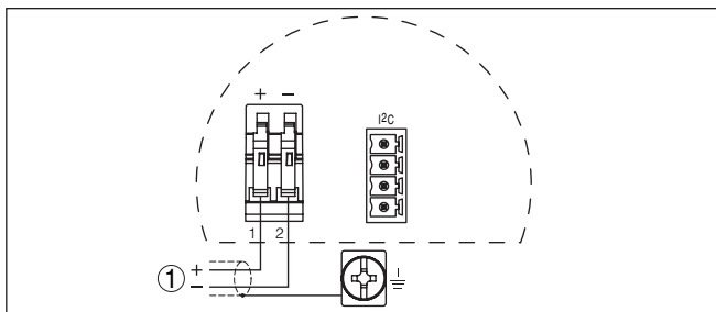
Fig. 6: Schéma de raccordement - boîtier à deux chambres
