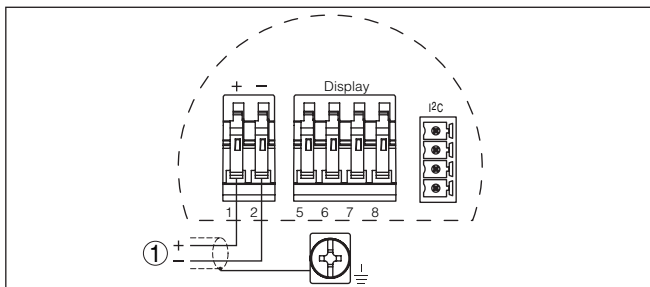
Fig. 5: Schéma de raccordement - boîtier à chambre unique
