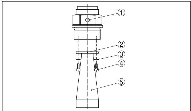
Fig. 1: Démontage de l'antenne cône
