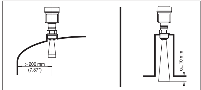
Fig. 3: Écarts de l'antenne à la paroi de la cuve/au couvercle de la cuve
