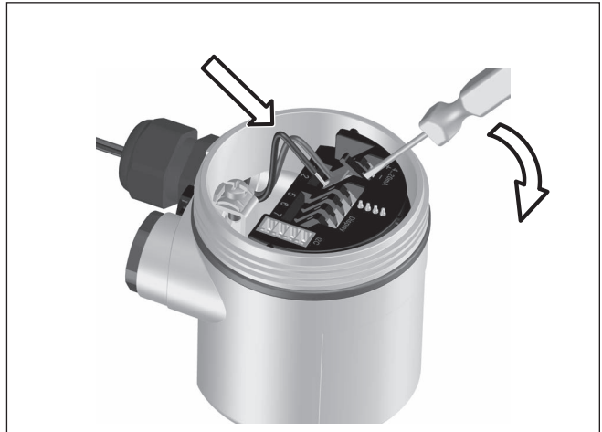
Fig. 4: Étapes de raccordement 6 et 7
