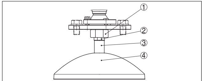
Fig. 2: Démontage de l'antenne parabolique
