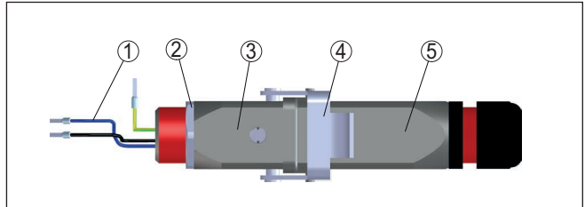
插图. 1: 插接器的构造 Harting HAN 8D - 举例
