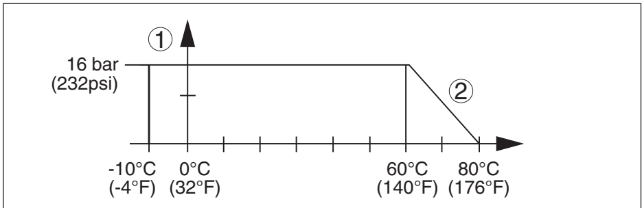
Fig. 26: Pression process - température process - VEGACAP 35 avec raccord process en 316L
