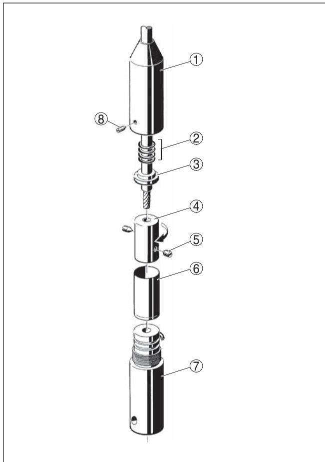
Fig. 24: Raccourcissement de la sonde câble
