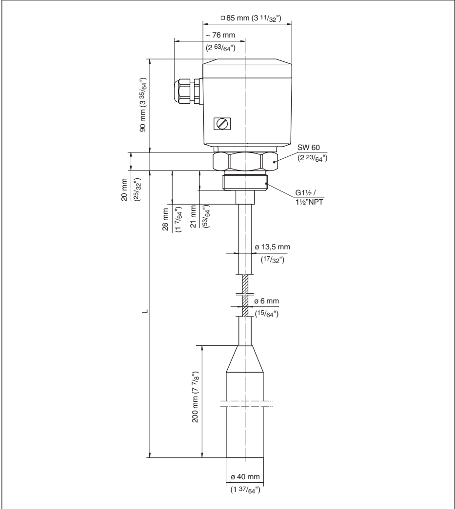
Fig. 28: VEGACAP 35, version câble avec \phi 6 \text{ mm} , version fileté G1\frac{1}{2} (ISO 228 T1)
