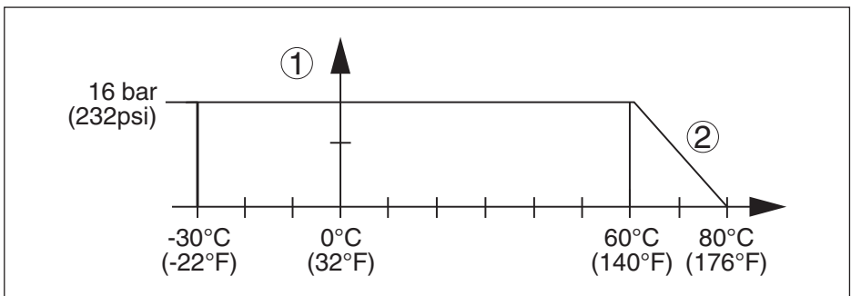
Fig. 27: Pression process - température process - VEGACAP 35 avec raccord process en 316Ti
