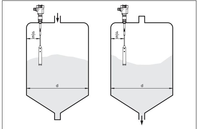
Fig. 5: Remplissage et vidange au centre
