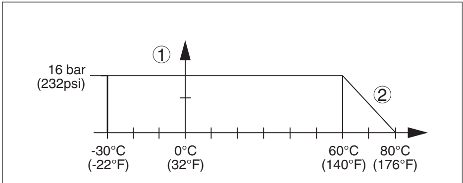
Fig. 25: Pression process - température process - VEGACAP 35 avec raccord process en aluminium
