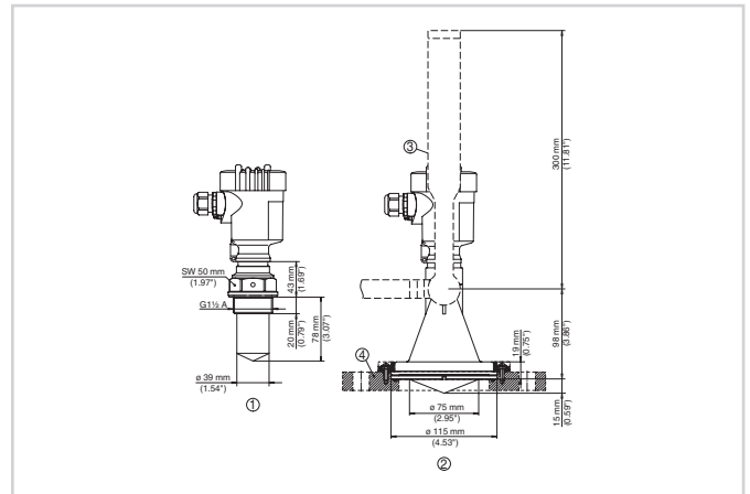
Afmetingen VEGAPULS 61
