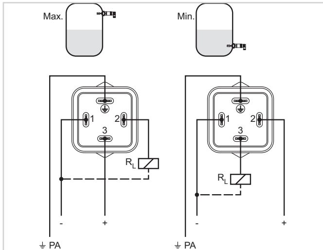
VEGASWING 51 met ventielstekker conform ISO 4400
