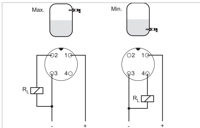
VEGASWING 51 met M12 x 1-connector
