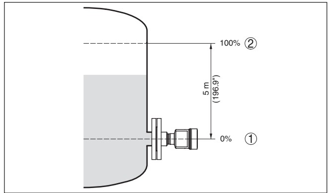
Fig. 9: Ejemplo de parametrización ajuste mín./máx. medición de nivel
