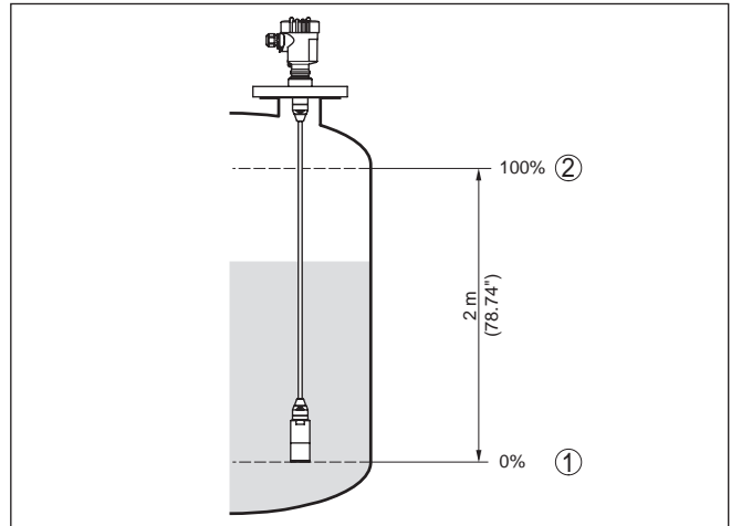
Fig. 6: Exemple de paramétrage réglage min./max. mesure de niveau
