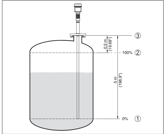
Fig. 6: Exemple de paramétrage réglage min./max.
