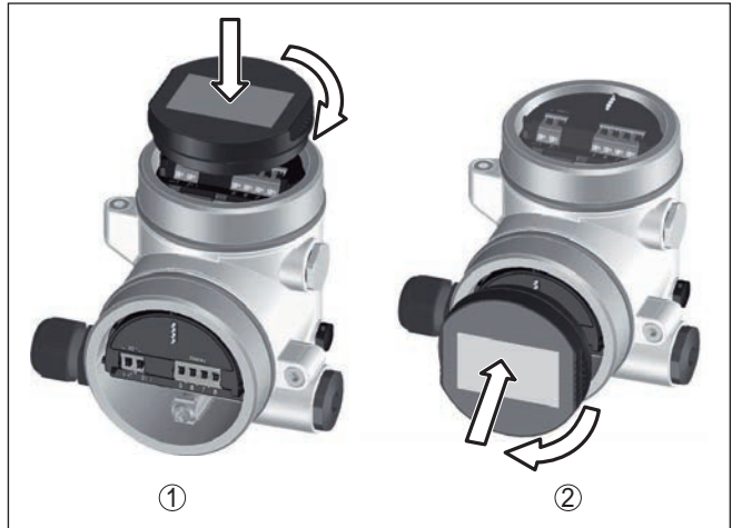
Fig. 5: Montage du module d'affichage et de réglage dans le boîtier à deux chambres
