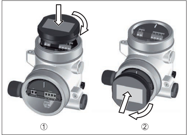
Fig. 6: Montage du module d'affichage et de réglage dans le boîtier à deux chambres
