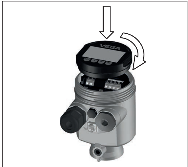
Fig. 5: Montage du module d'affichage et de réglage dans le boîtier à chambre unique se trouvant dans le compartiment de l'électronique
