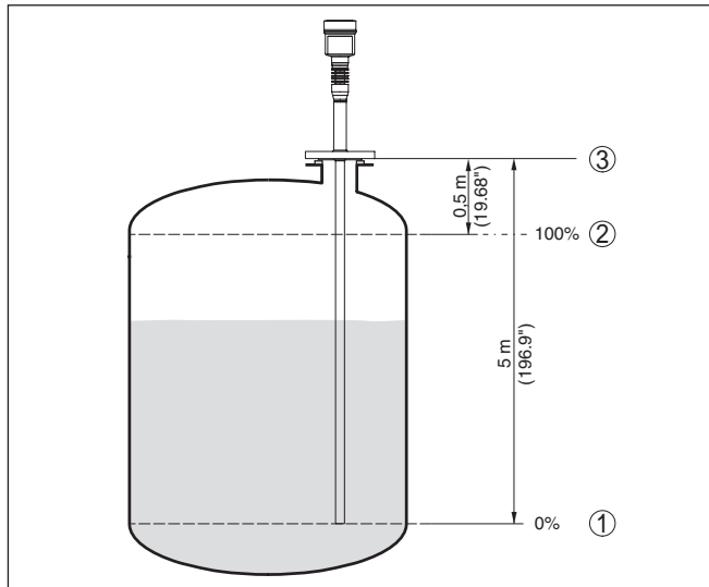
Fig. 7: Exemple de paramétrage réglage min./max.
