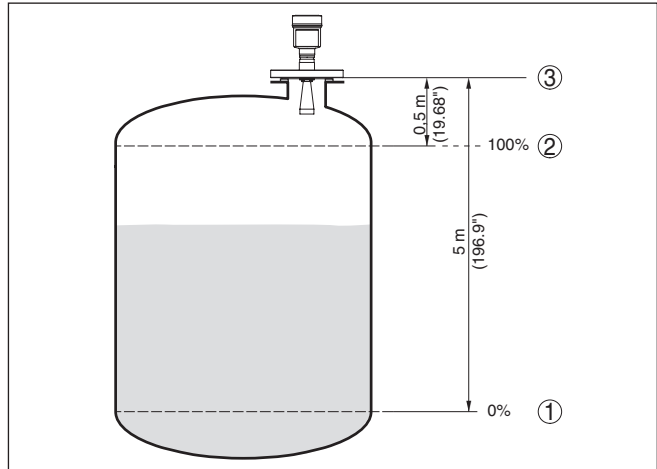
Fig. 10: Exemple de paramétrage réglage min./max.
