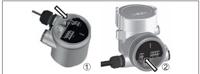
Fig. 5: Étapes de raccordement 5 et 6
