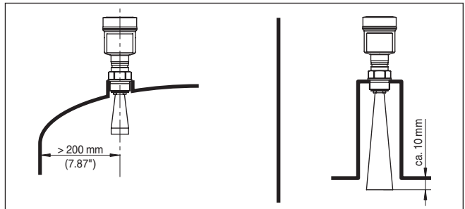
Fig. 4: Écarts de l'antenne à la paroi de la cuve/au couvercle de la cuve
