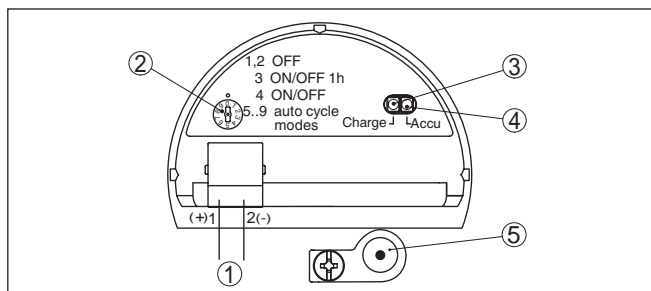
Figura 3: Vano di alimentazione
