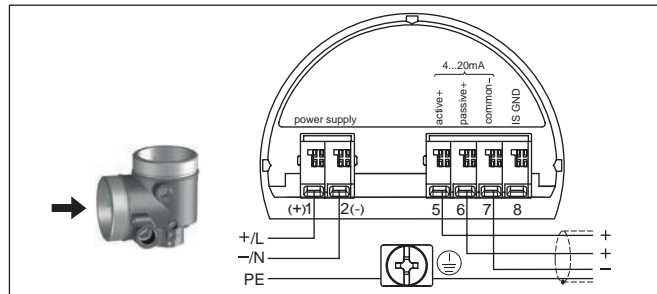
Fig. 3: Compartiment de raccordement boîtier deux chambres pour tension de réseau
