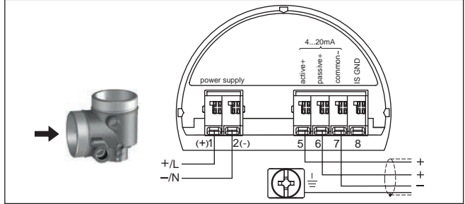
Fig. 4: Compartiment de raccordement boîtier deux chambres pour très basse tension
