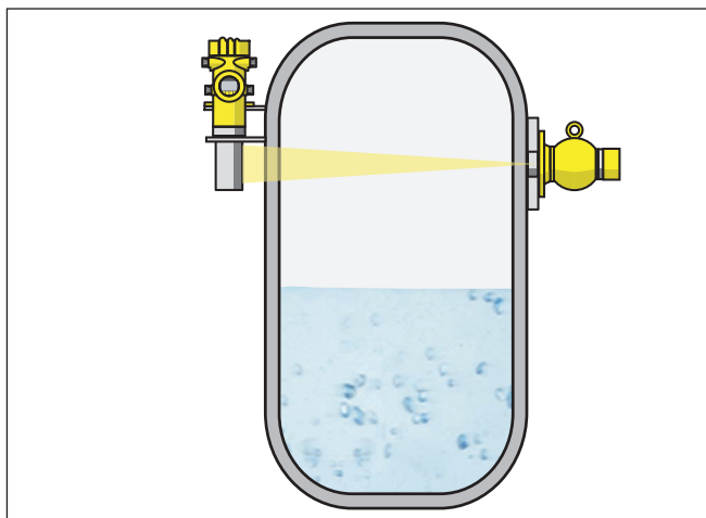
Fig. 6: POINTRAC 31 als maximaal niveausignalering (niet bedekt)
