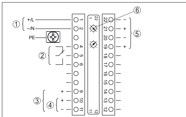
Fig. 10: Elektronica- en aansluitruimte bij niet-Ex instrumenten en instrumenten met niet-intrinsiekveilige stroomuitgang
