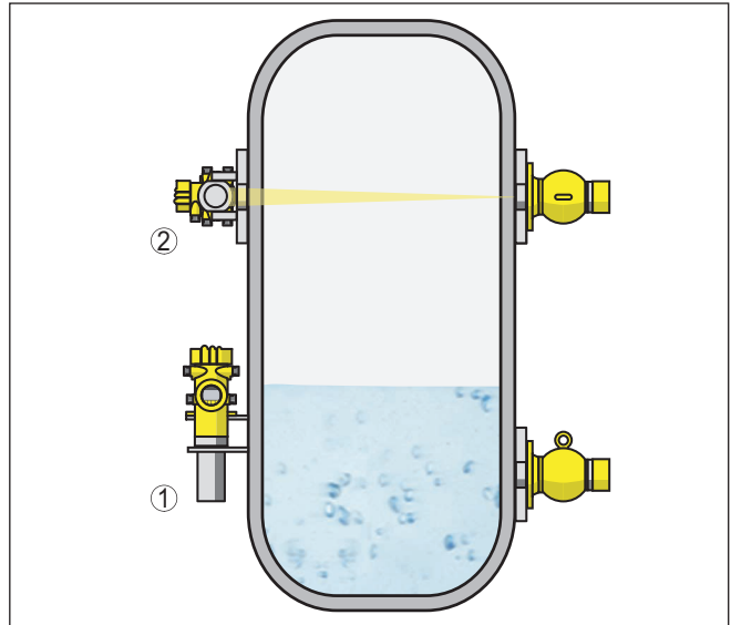
Fig. 3: Montagepositie - niveaudetectie - uitvoering met detectorbuis
