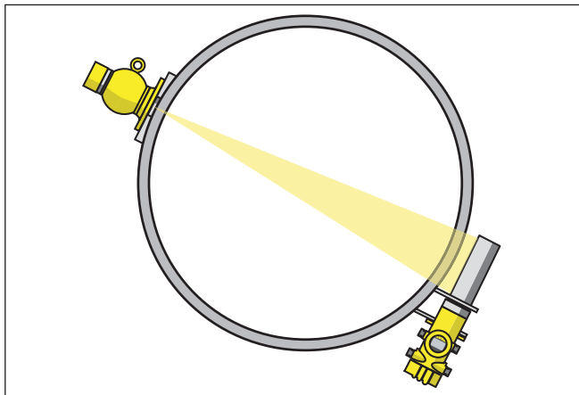
Fig. 8: POINTRAC 31 als niveausignalering (bovenaanzicht)
