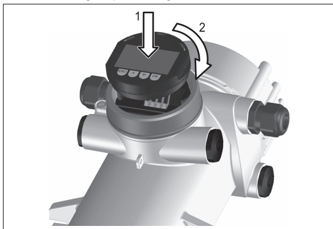
Fig. 14: Aanwijs- en bedieningsmodule inzetten
