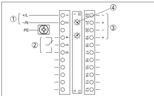
Fig. 12: Elektronica- en aansluitruimte (Ex-d) bij instrumenten met intrinsiekveilige stroomuitgang
