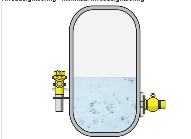
Fig. 7: POINTRAC 31 als minimaal niveausignalering (bedekt)
