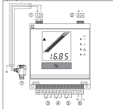
Abb. 19: Schéma de raccordement avec capteur bifilaire
