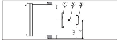
Abb. 18: Montage sur rail
