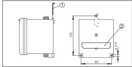
Abb. 17: Fixation par vis
