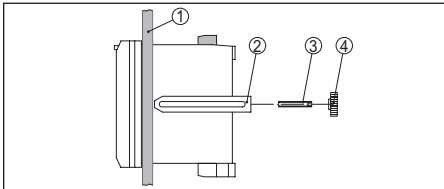
Abb. 16: Montage encastré
