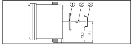
Abb. 4: Tragschienenmontage
