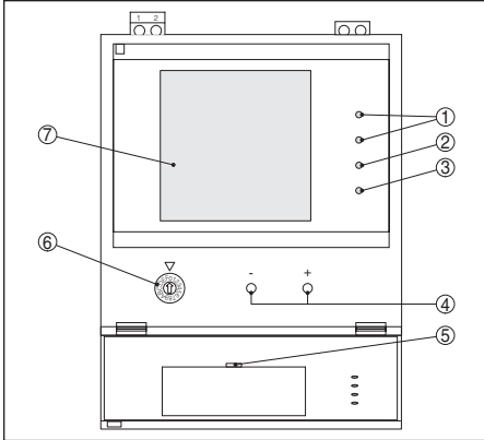
Abb. 15: VEGAMET 381 Ex
