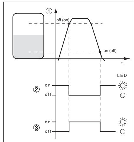
Abb. 28: Modos del relé
