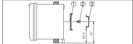
Abb. 25: Montaje en regleta
