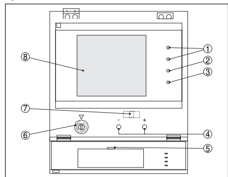
Abb. 27: Elementos de indicación y ajuste
