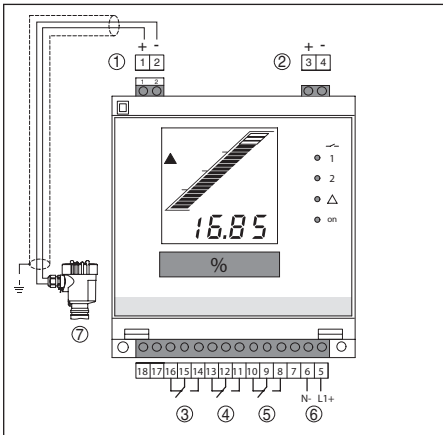
Abb. 26: Esquema de conexión con sensor de dos hilos
