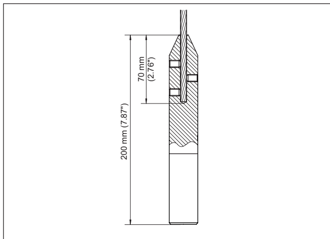
Figura 25: Tenete conto del peso tenditore ed accorciate la fune in proporzione.
