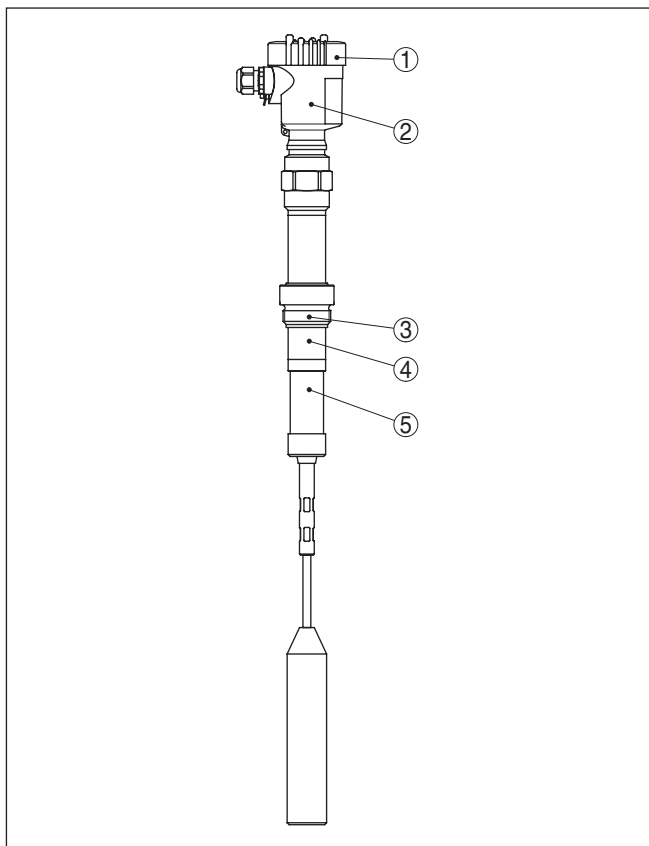
Figura 1: VEGACAL 67 con custodia di resina
