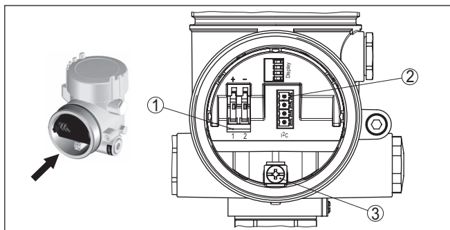
Figura 13: Vano di allacciamento - custodia a due camere
