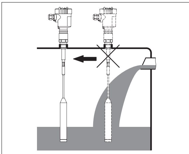
Figura 6: Prodotto in ingresso
