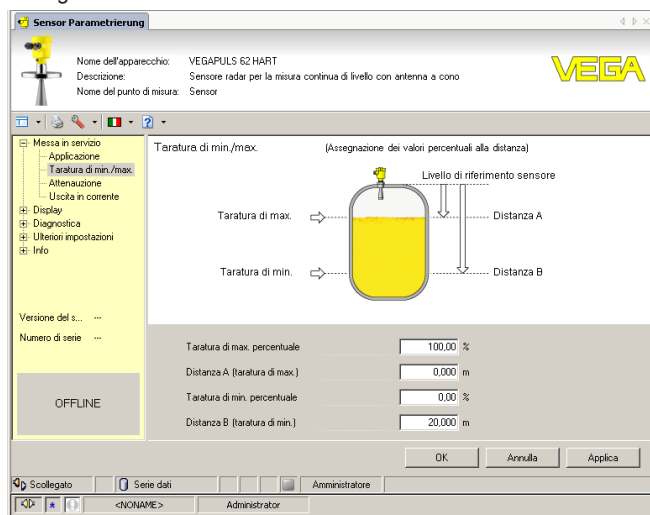
Figura 21: Esempio di una maschera DTM
