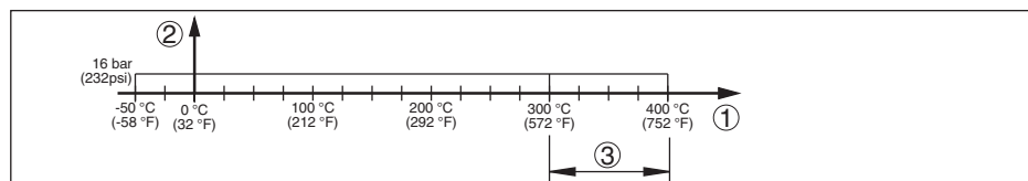
Figura 26: Temperatura di processo - Pressione di processo
