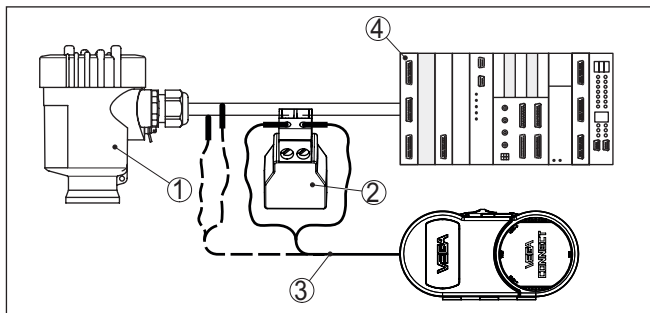
Figura 20: Collegamento del PC via HART alla linea del segnale
