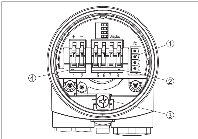
Figura 9: Vano dell'elettronica e di connessione - custodia a una camera
