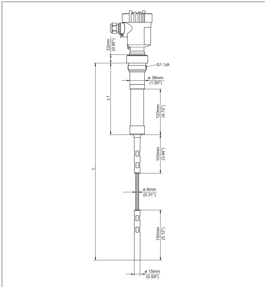
Figura 31: VEGACAL 67, sonda di misura a fune con isolamento in ceramica con puntale a crimpare / -50 ... +350 °C 8)
