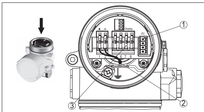
Figura 12: Vano dell'elettronica - custodia a due camere
