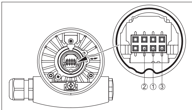
Figura 24: Controllare la resistenza all'interno della sonda di misura
