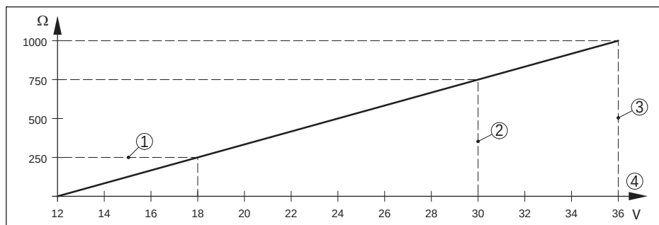
Figura 27: Diagramma della tensione
