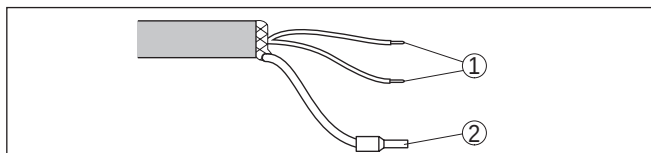
Figura 15: Assegnazione dei conduttori del cavo di collegamento
