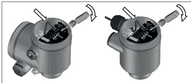
Figura 7: Operazioni di collegamento 6 e 7
