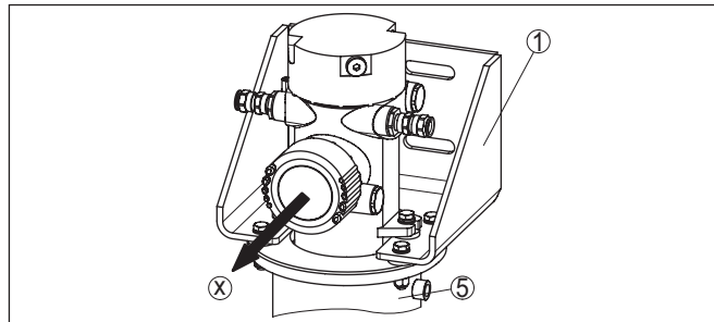
Abb. 4: Montagerichtung des Sensors zum Befestigungswinkel
