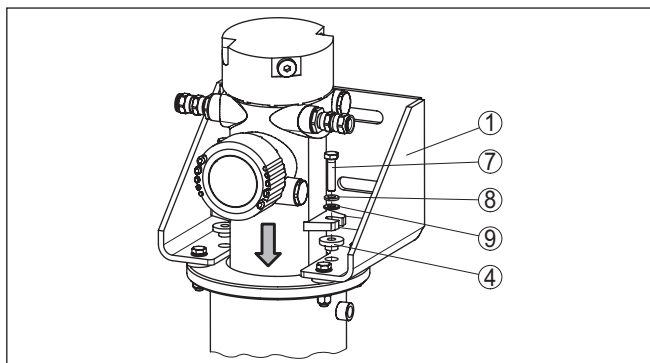
Abb. 5: Montage des Sensors
