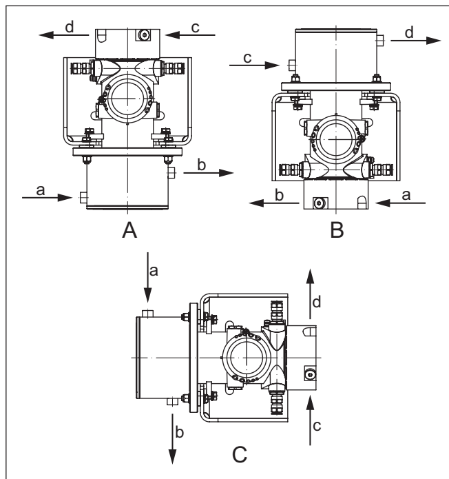
Abb. 7: Montagestellung des Kühlsystems - Fließrichtung des Kühlmittels (a, b, c ...) beachten
