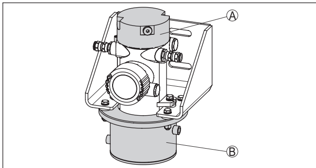
Abb. 1: Aktives Wasser-Kühlsystem mit Befestigungswinkel (optional)
