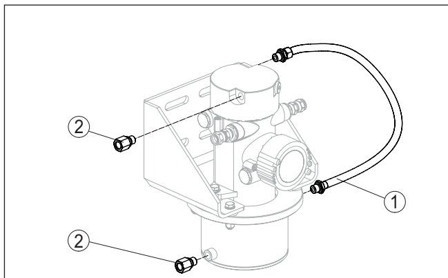
Abb. 10: Szintillatorkühlung - Schläuche und Adapter
