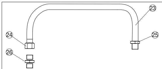
Fig. 16: Prefab koelmiddelslang
