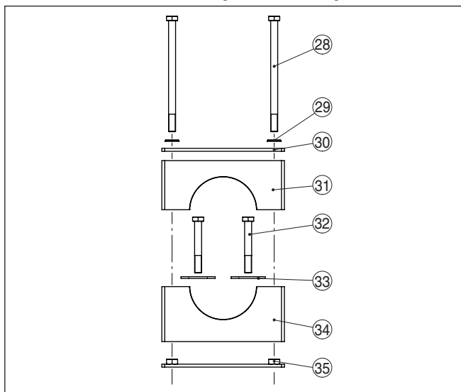
Fig. 10: Montageklemmen
