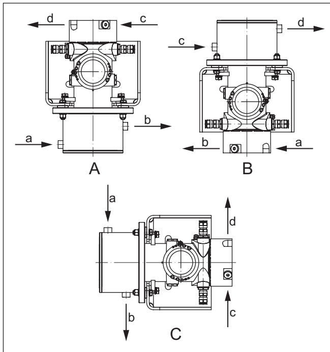
Fig. 13: Montagepositie van het koelsysteem - doorstroomrichting van het koelmiddel (a, b, c ...) aanhouden
