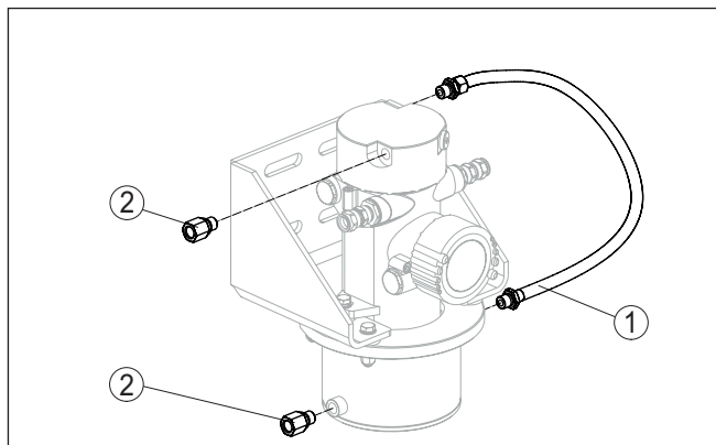
Fig. 18: Scintillatorkoeling - slangen en adapters
