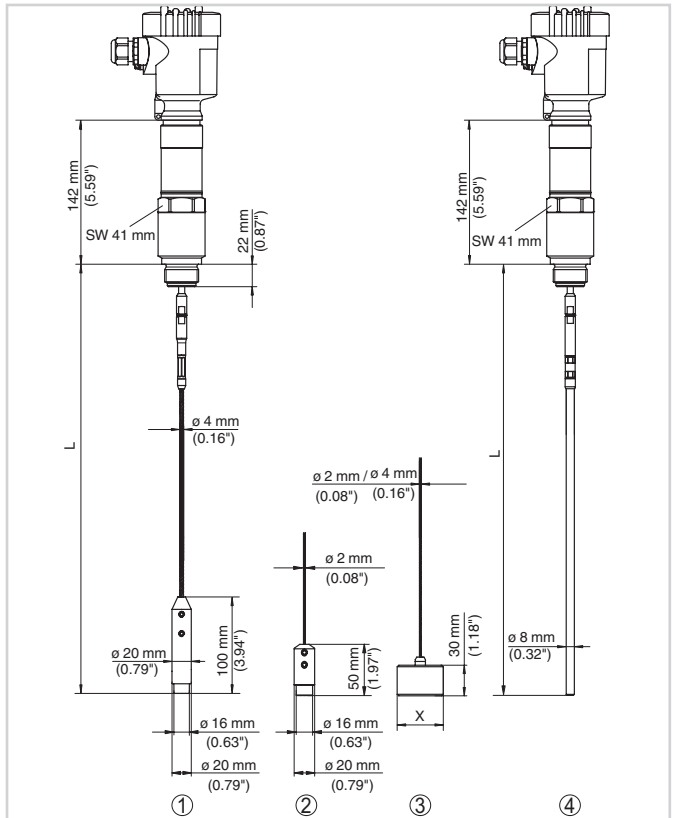
VEGAFLEX 86 - schroefdraaduitvoering (-20 ... +250 °C)
