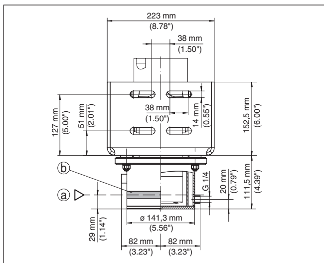
Fig. 5: Positie van de sensormarkering en boorplan van de bevestigingsbeugel - POINTRAC 31 - korte uitvoering (46 mm)
