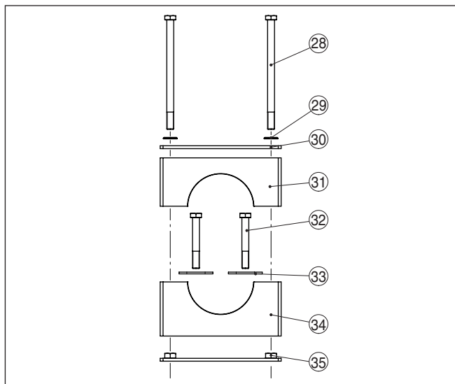
Fig. 10: Montageklemmen
