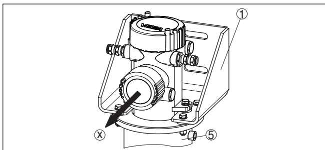
Fig. 6: Montagerichting van de sensor ten opzichte van de bevestigingsbeugel
