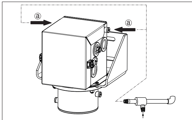
Fig. 15: Aansluiting van het koelluchtsysteem (wervelstroomkoeler) - POINTRAC 31 - korte uitvoering (46 mm)
