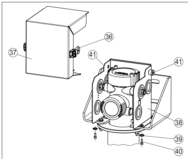
Fig. 11: Montage van de behuizingskoelbox
