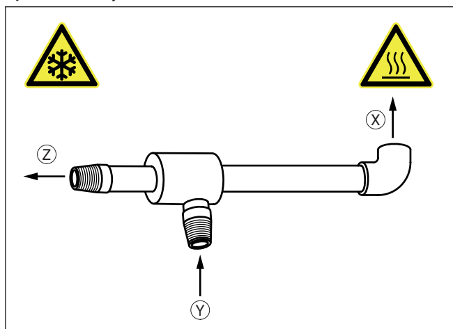
Fig. 13: Wervelstroomkoeler (vortex-koeler)
