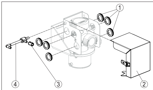
Fig. 17: Reservedelen - luchtkoeling POINTRAC - korte uitvoering (46 mm)
