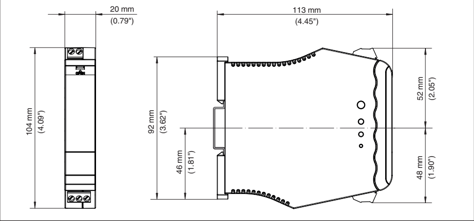
Figura 2: Dimensioni VEGATRENN 151
