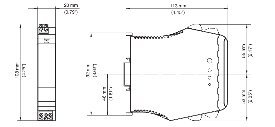
Figura 2: Dimensioni VEGATRENN 152
