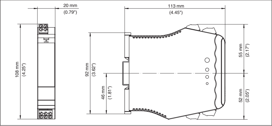
Fig. 2: Afmetingen VEGATRENN 152
