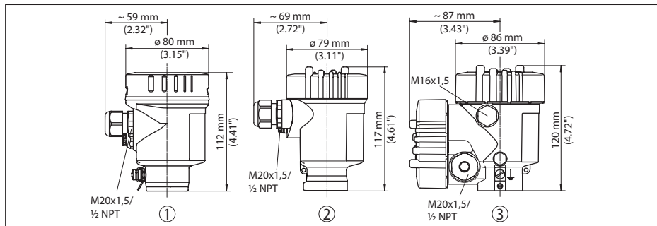
Fig. 55: Huisuitvoeringen in beschermingsklasse IP66/IP68 (0,2 bar), (met ingebouwde display- en bedieningsmodule wordt het huis 18 mm hoger)
