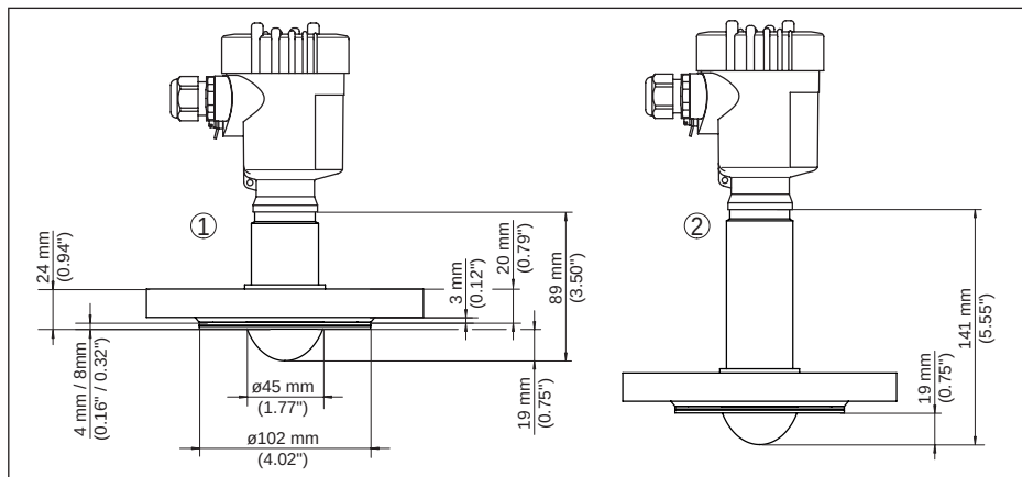
Fig. 63: VEGAPULS 64, gekapseld antennesysteem DN 50 PN 40
