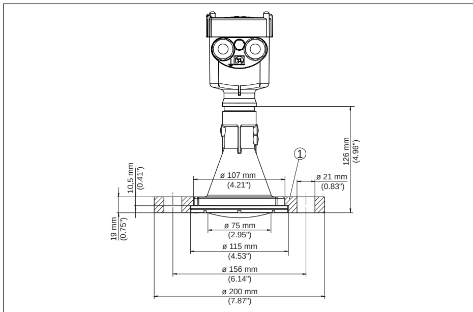
Fig. 57: Radarsensor met overschuifflens passend voor 3" 150 lbs, DN 80 PN 16
