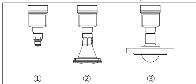
Fig. 2: Antennesystemen VEGAPULS 64
