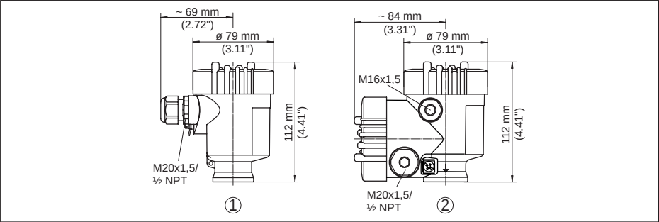
Fig. 52: Huisuitvoeringen in beschermingsklasse IP66/IP67 (met ingebouwde aanwijs- en bedieningsmodule wordt het huis 9 mm hoger)
