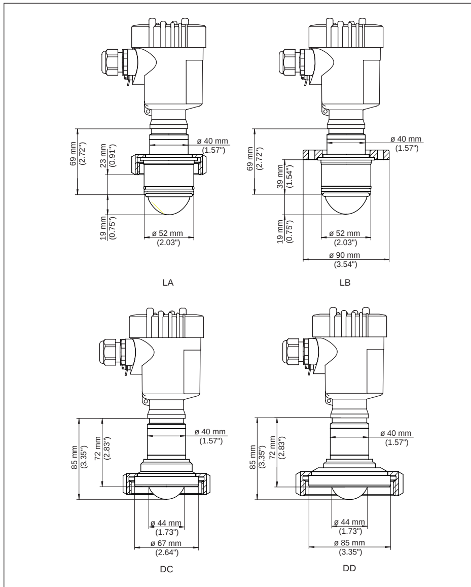
Fig. 67: VEGAPULS 64, hygiënische aansluiting met ingekapseld antennesysteem
