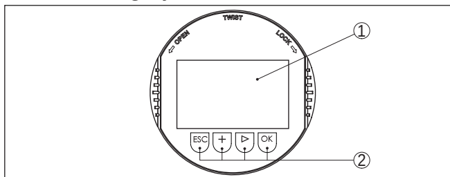
Fig. 36: Aanwijs- en bedieningselementen
