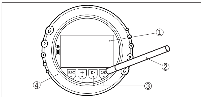
Fig. 37: Display- en bedieningselement - met bediening via magneetpen
