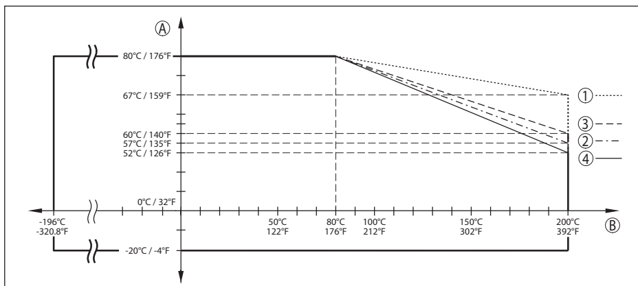
Fig. 51: Derating omgevingstemperatuur, flens DN 50/2" en DN 80/3" met gekapseld antennesysteem tot -196 ... +200 °C (-320.8 ... +392 °F)
