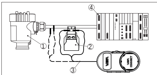
Fig. 40: Aansluiting van de PC via HART op de signaalkabel
