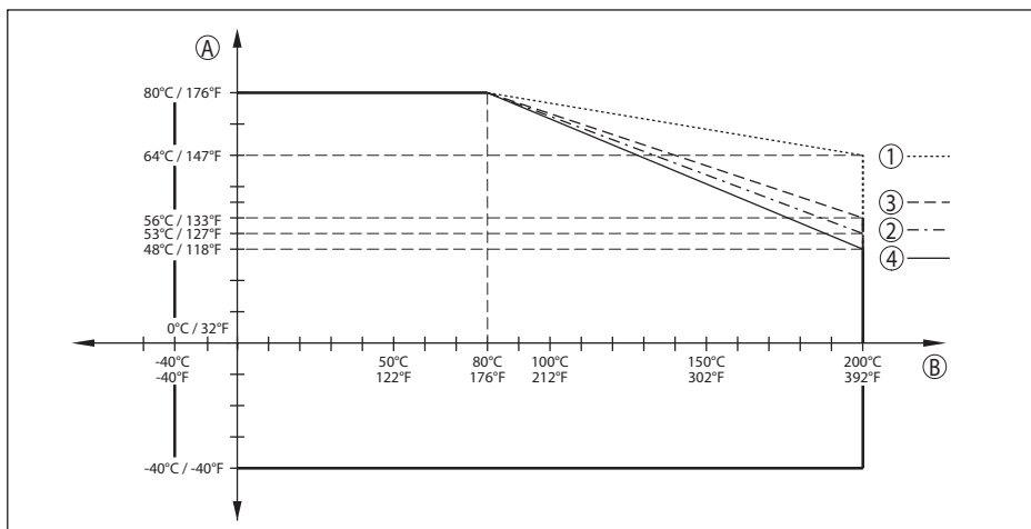
Fig. 47: Derating omgevingtemperatuur, schroefdraad G \frac{3}{4} en G1 \frac{1}{2} met geïntegreerde hoornantenne tot +200 °C (+392 °F)
