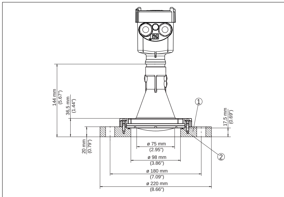
Fig. 59: Radarsensor met adapterflens DN 100 PN 6
