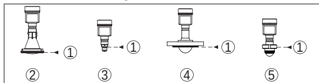
Fig. 14: Positie van het referentievlak
