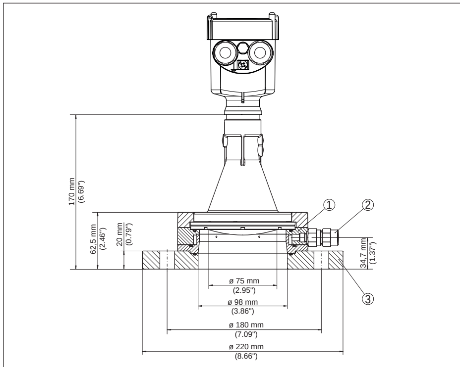
Fig. 60: VEGAPULS 64, adapterflens en spoelaansluiting DN 100 PN 6
