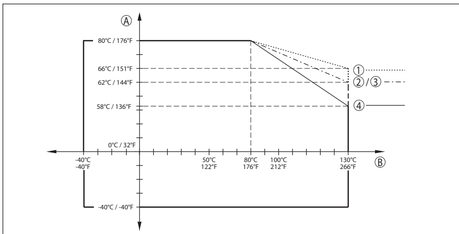
Fig. 49: Derating omgevingstemperatuur, flens DN 50/2" en DN 80/3" met gekapseld antennesysteem tot +130 °C (+266 °F)
