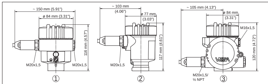
Fig. 56: Huisuitvoeringen in beschermingsklasse IP66/IP68 (1 bar), (met ingebouwde display- en bedieningsmodule wordt het huis 18 mm/0.71 in hoger)
