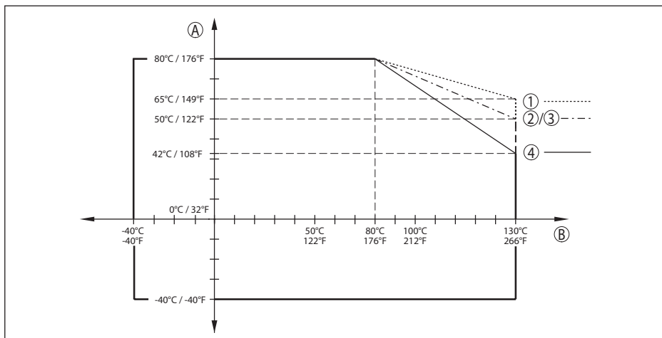
Fig. 46: Derating omgevingtemperatuur, schroefdraad G \frac{3}{4} en G1 \frac{1}{2} met geïntegreerde hoornantenne tot +130 °C (+266 °F)
