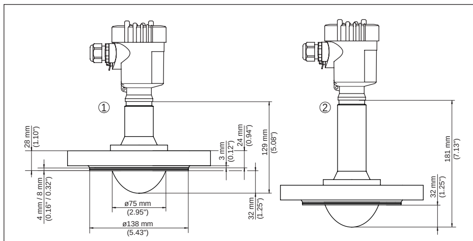
Fig. 64: VEGAPULS 64, gekapseld antennesysteem DN 80 PN 40
