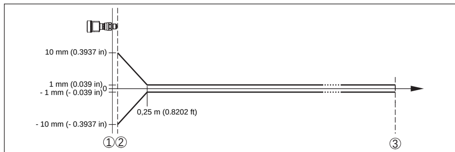
Fig. 45: Meetafwijking onder referentieomstandigheden (voorbeeld schroefdraad met geïntegreerde hoornantenne, geldt overeenkomstig voor alle uitvoeringen) 9)
