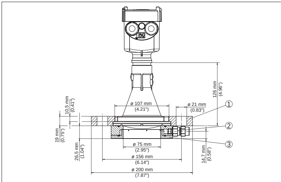
Fig. 58: Radarsensor met overschuifflens en spoelaansluiting passend voor 3" 150 lbs, DN 80 PN 16
