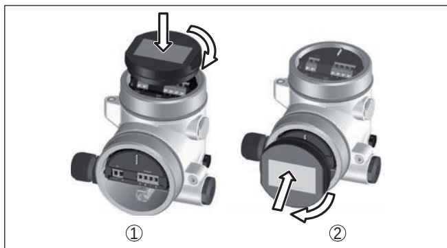
Fig. 35: Plaatsen van de display- en bedieningsmodule bij de tweekamerbehuizing
