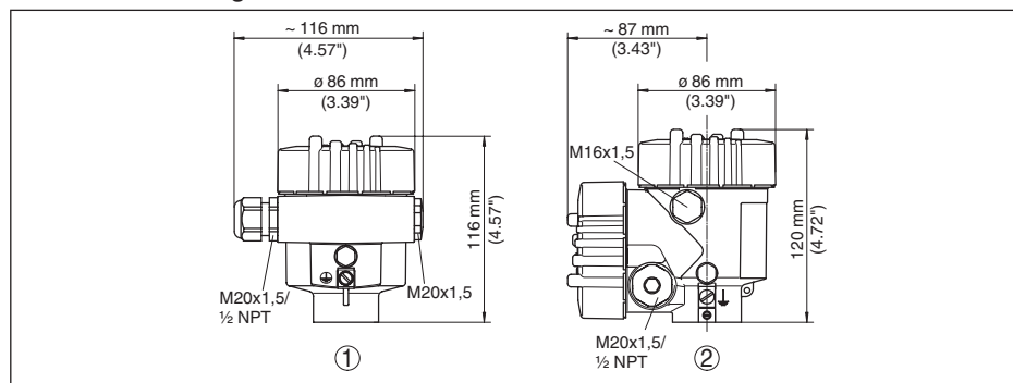
Fig. 53: Huisuitvoeringen in beschermingsklasse IP66/IP68 (0,2 bar), (met ingebouwde display- en bedieningsmodule wordt het huis 18 mm hoger)
