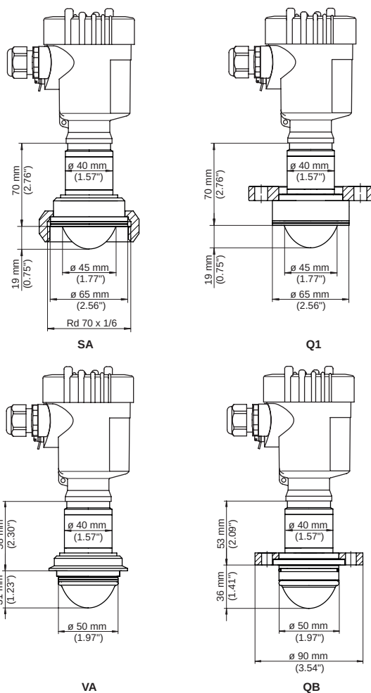
Fig. 66: VEGAPULS 64, hygiënische aansluiting met ingekapseld antennesysteem
