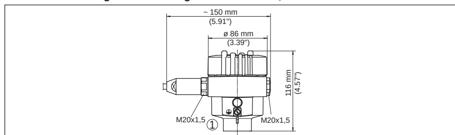
Fig. 54: Huisuitvoeringen in beschermingsklasse IP66/IP68 (1 bar), (met ingebouwde display- en bedieningsmodule wordt het huis 18 mm/0.71 in hoger)
