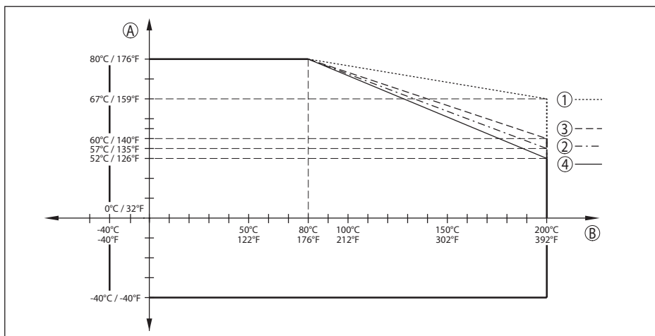
Fig. 50: Derating omgevingstemperatuur, flens DN 50/2" en DN 80/3" met gekapseld antennesysteem tot +200 °C (+392 °F)
