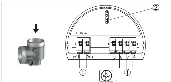
Fig. 30: Elektronicaruimte - tweekamerbehuizing
