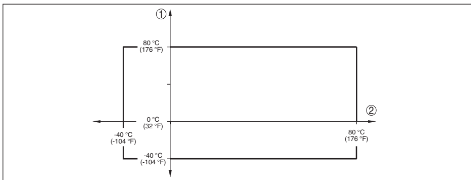
Fig. 48: Derating omgevingstemperatuur, kunststofhoornantenne
