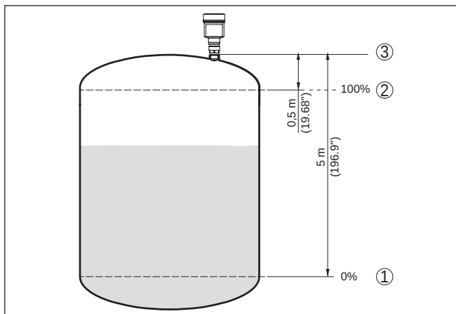
Fig. 38: Parametrevoorbeeld min.-/max.-inregeling
