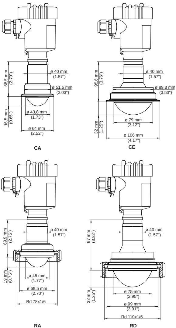
Fig. 65: VEGAPULS 64, hygiënische aansluiting met ingekapseld antennesysteem
