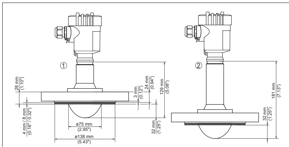
Fig. 67: VEGAPULS 64, gekapseld antennesysteem DN 80 PN 40
