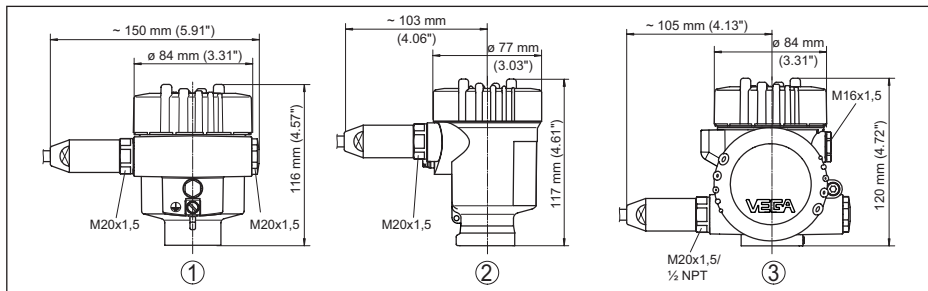
Fig. 59: Huisuitvoeringen in beschermingsklasse IP66/IP68 (1 bar), (met ingebouwde display- en bedieningsmodule wordt het huis 18 mm/0.71 in hoger)
