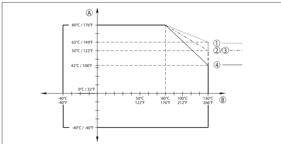
Fig. 49: Derating omgevingstemperatuur, schroefdraad G \frac{3}{4} en G1 \frac{1}{2} met geïntegreerde hoornantenne tot +130 °C (+266 °F)
