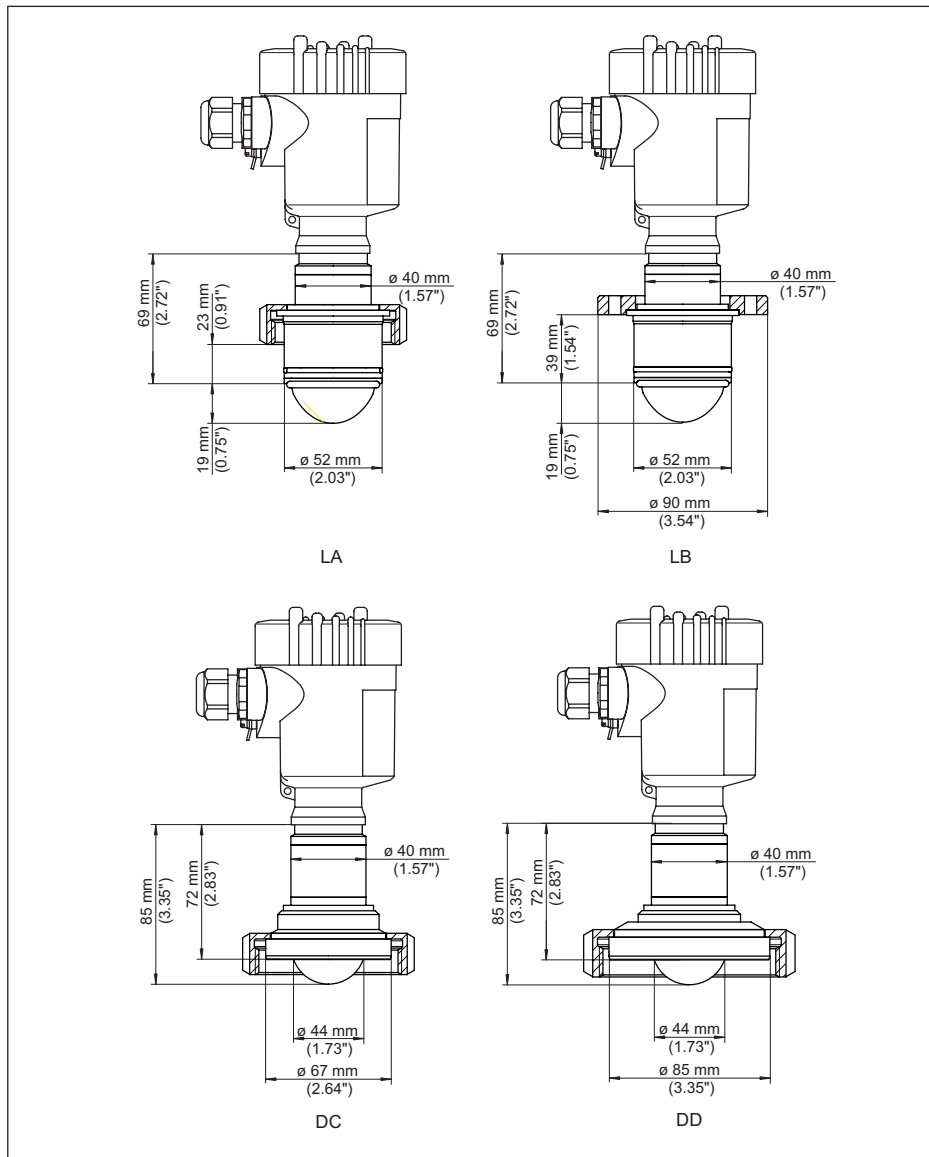
Fig. 70: VEGAPULS 64, hygiënische aansluiting met ingekapseld antennesysteem
