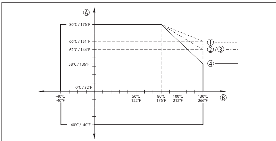
Fig. 52: Derating omgevingtemperatuur, flens DN 50/2" en DN 80/3" met gekapseld antennesysteem tot +130 °C (+266 °F)
