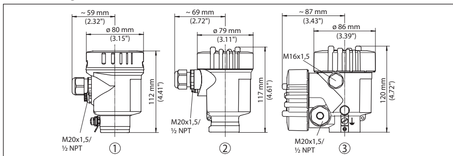
Fig. 58: Huisuitvoeringen in beschermingsklasse IP66/IP68 (0,2 bar), (met ingebouwde display- en bedieningsmodule wordt het huis 18 mm hoger)
