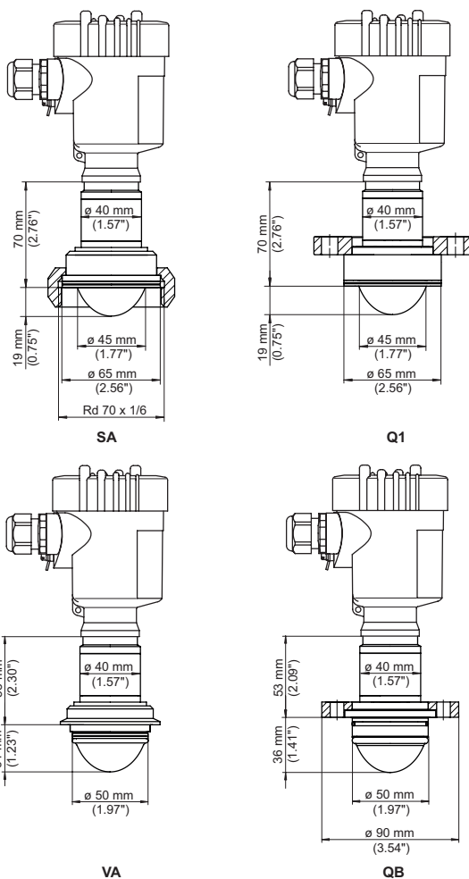
Fig. 69: VEGAPULS 64, hygiënische aansluiting met ingekapseld antennesysteem
