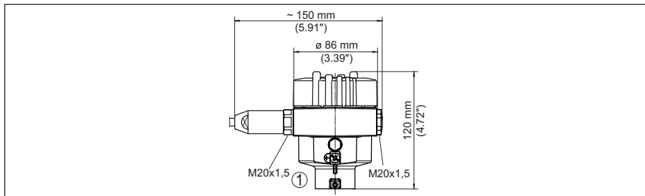
Fig. 57: Huisuitvoeringen in beschermingsklasse IP66/IP68 (1 bar), (met ingebouwde display- en bedieningsmodule wordt het huis 18 mm/0.71 in hoger)
