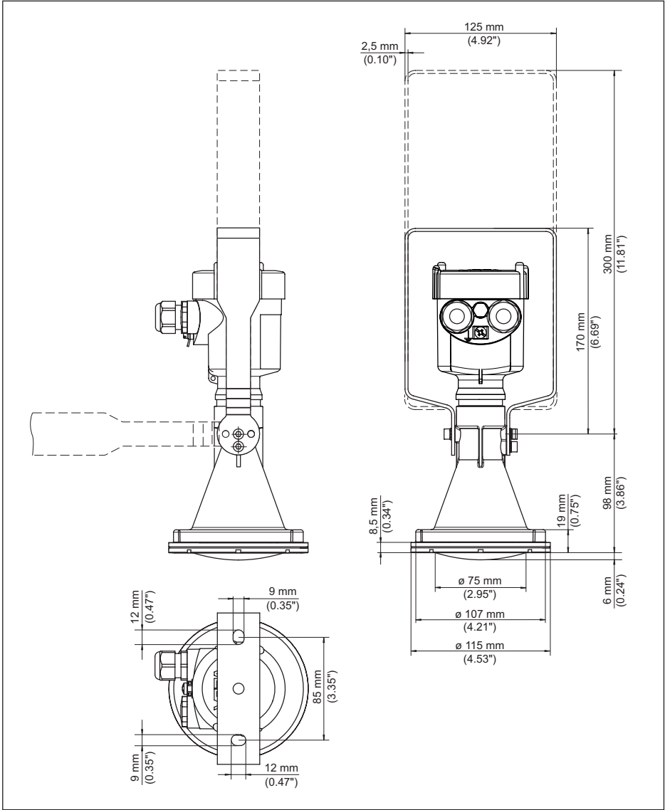
Fig. 64: VEGAPULS 64, kunststofhoornantenne, montagebeugel in 170 of 300 mm lengte
