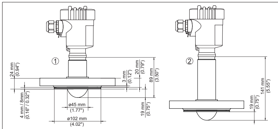
Fig. 66: VEGAPULS 64, gekapseld antennesysteem DN 50 PN 40
