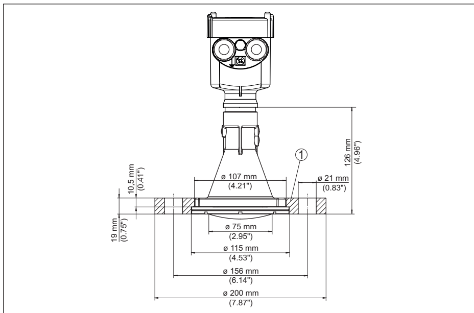
Fig. 60: Radarsensor met overschuifflens passend voor 3" 150 lbs, DN 80 PN 16
