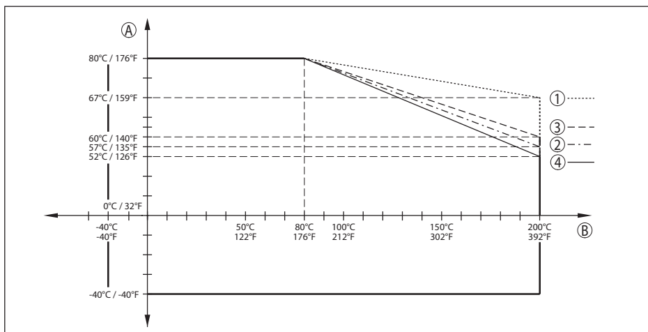
Fig. 53: Derating omgevingstemperatuur, flens DN 50/2" en DN 80/3" met gekapseld antennesysteem tot +200 °C (+392 °F)
