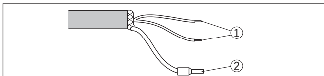
Fig. 36: Aderbezetting vast aangesloten aansluitkabel
