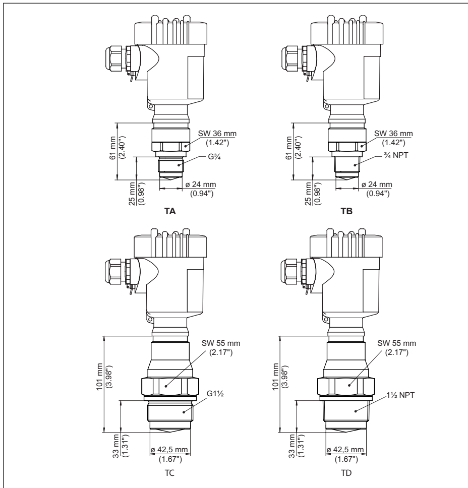
Fig. 65: VEGAPULS 64, schroefdraad met geïntegreerde hoornantenne
