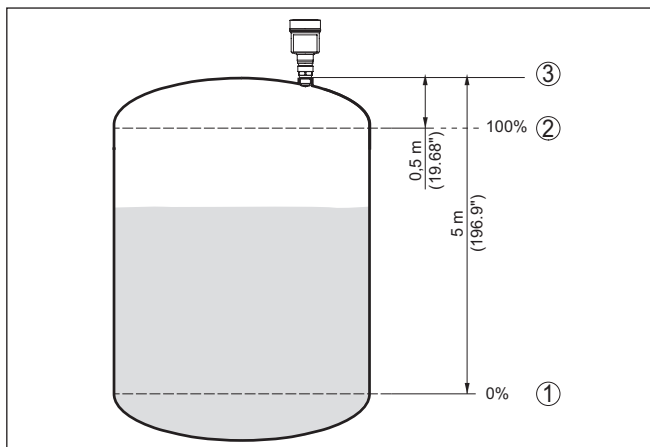
Fig. 41: Parametrevoorbeeld min.-/max.-inregeling
