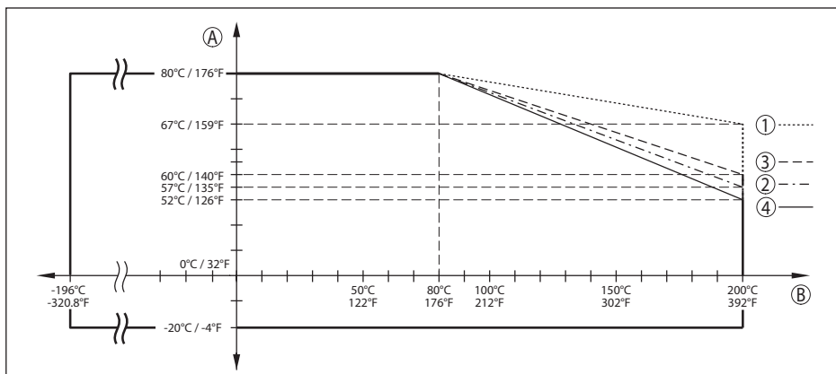
Fig. 54: Derating omgevingstemperatuur, flens DN 50/2" en DN 80/3" met gekapseld antennesysteem tot -196 ... +200 °C (-320.8 ... +392 °F)
