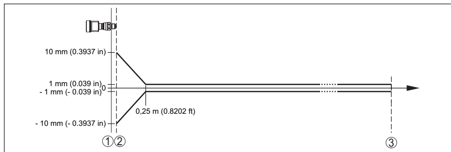
Fig. 48: Meetafwijking onder referentieomstandigheden (voorbeeld schroefdraad met geïntegreerde hoornantenne, geldt overeenkomstig voor alle uitvoeringen) 8)
