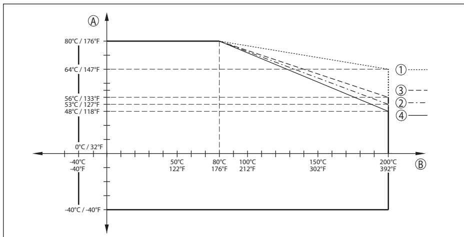
Fig. 50: Derating omgevingstemperatuur, schroefdraad G \frac{3}{4} en G1 \frac{1}{2} met geïntegreerde hoornantenne tot +200 °C (+392 °F)
