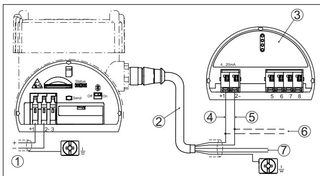
Fig. 35: Aansluiting voedingsspanning en plics®-sensor
