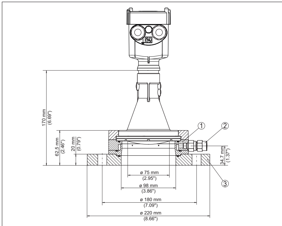
Fig. 63: VEGAPULS 64, adapterflens en spoelaansluiting DN 100 PN 6
