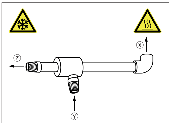
Fig. 9: Wervelstroomkoeler (vortex-koeler)
