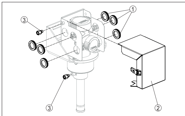
Fig. 13: Reservedelen - luchtkoeling met persluchtaansluiting (werkplaats) - scintillatorkoeling met conduit-aansluiting
