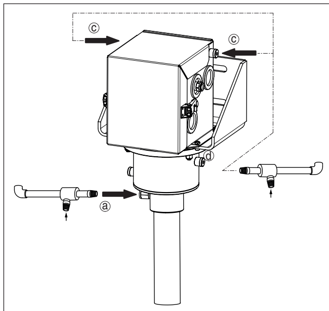
Fig. 10: Aansluiting van de koelluchtsystemen (wervelstroomkoeler)
