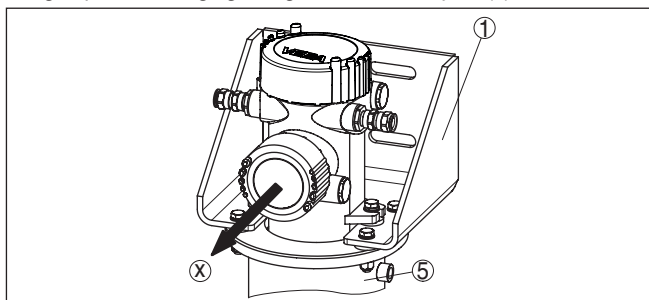
Fig. 3: Montagerichting van de sensor ten opzichte van de bevestigingsbeugel
