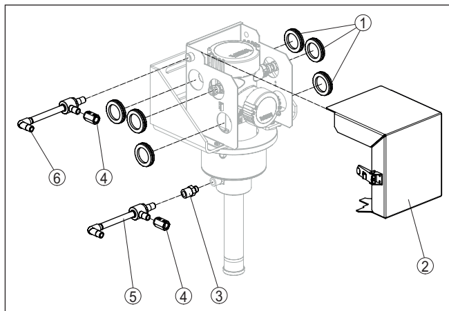
Fig. 12: Reservedelen - luchtkoeling met wervelstroomkoeler - scintillatorkoelbuis met conduit-aansluiting
