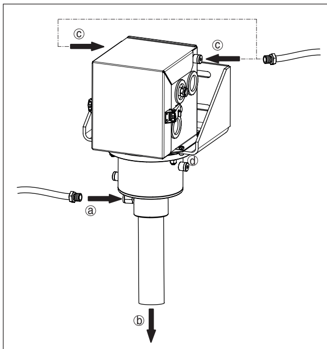
Fig. 11: Aansluiting van de koelluchtleidingen
