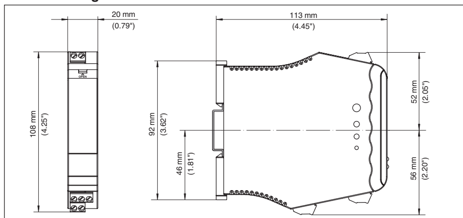
Fig. 2: Afmetingen VEGATRENN 141
