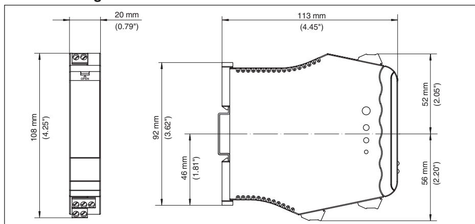
Fig. 2: Afmetingen VEGATRENN 141
