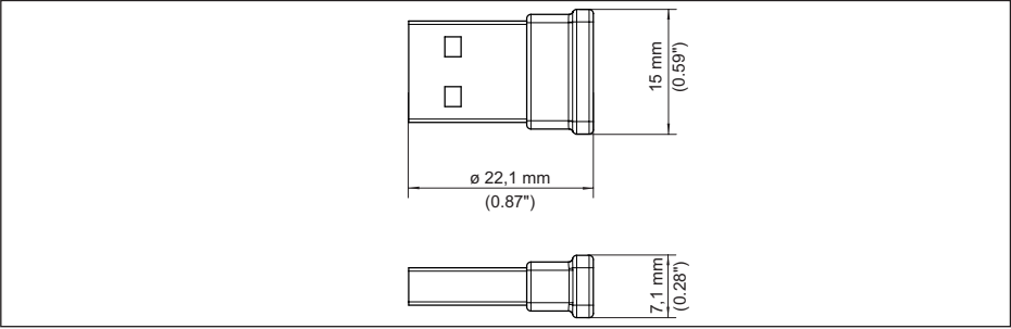
插图. 3: 蓝牙USB适配器的尺寸
