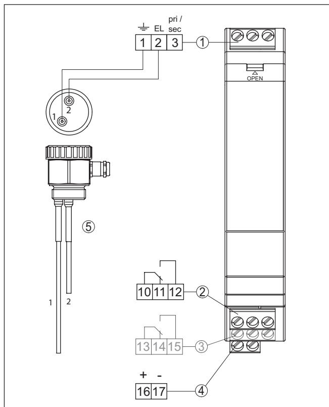
Fig. 1: Aansluitschema VEGATOR 131
