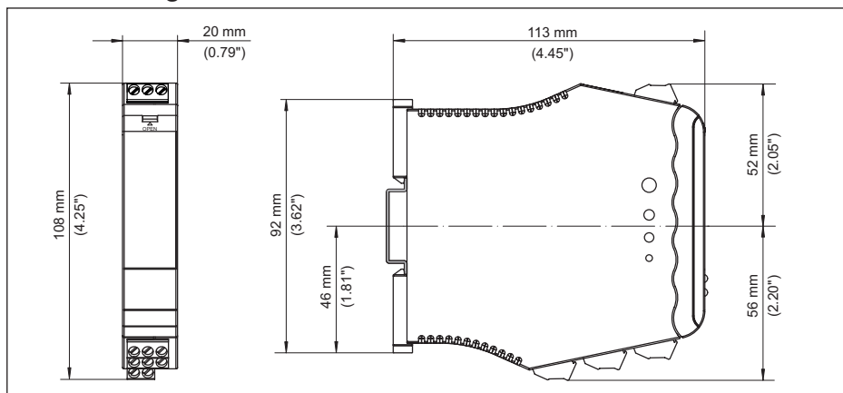
Fig. 7: Afmetingen VEGATOR 131
