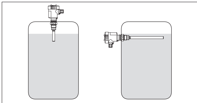
Fig. 5: Toepassingsvoorbeelden overloopbeveiliging met conductieve niveauschakelaar
