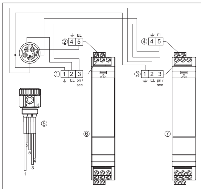
Fig. 2: Esquema de ligações VEGATOR 132
