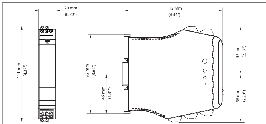
Fig. 8: Dimensões VEGATOR 132
