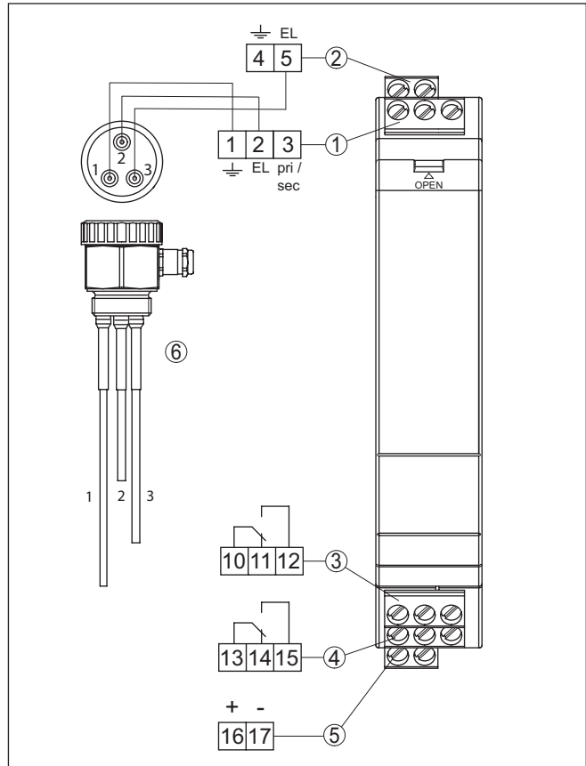
Fig. 1: Esquema de ligações VEGATOR 132
