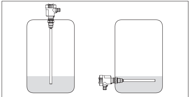
Fig. 7: Exemplos de aplicação proteção contra funciona- mento a seco com chave de nível condutiva
